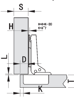
半盖门式 Half overlay
