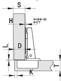
盖门式 Full overlay
